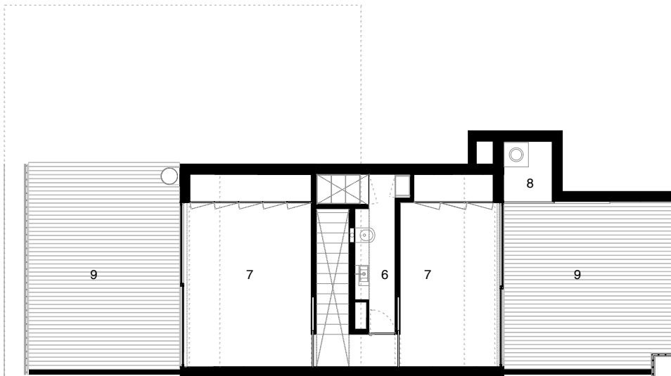
planta tipologia piso 1
