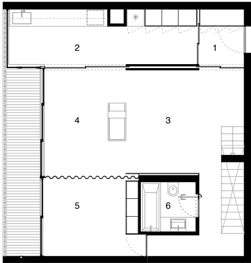
planta tipologia piso 0
