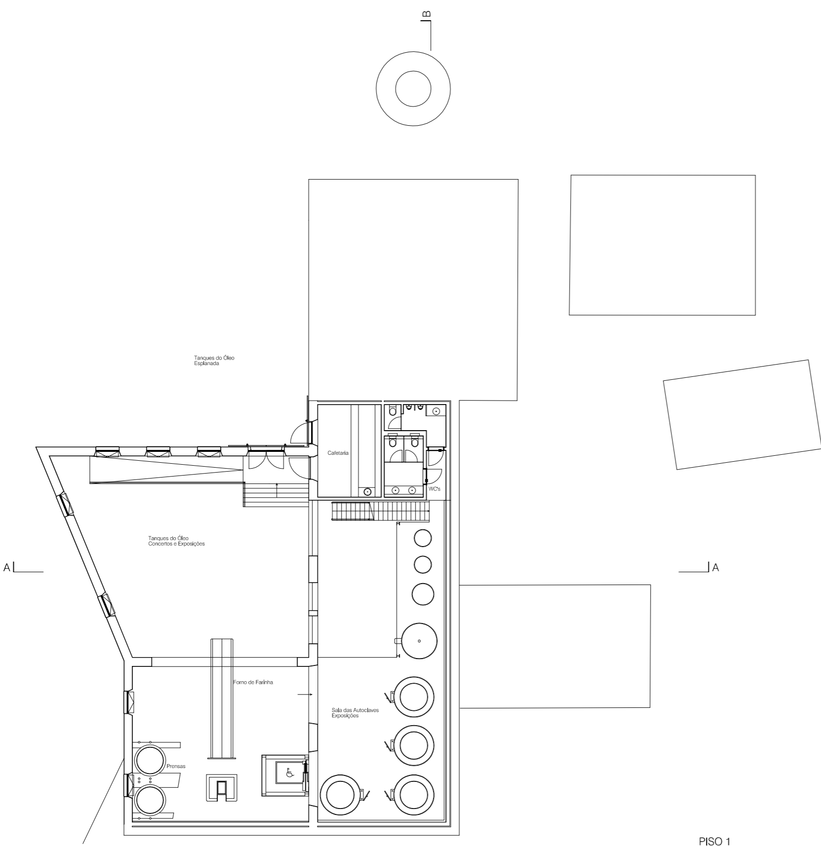
PISO 1
