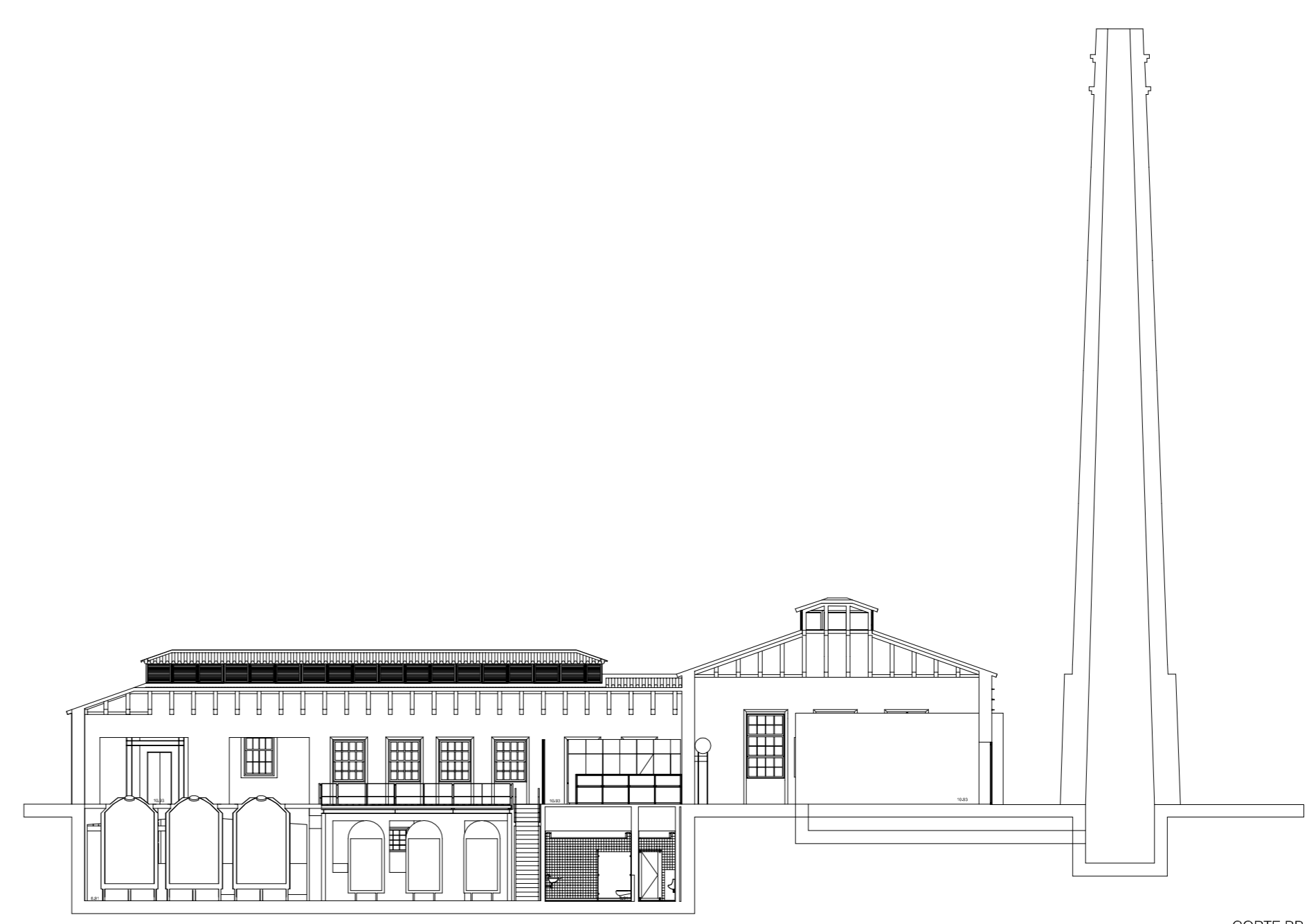
CORTE B-B
