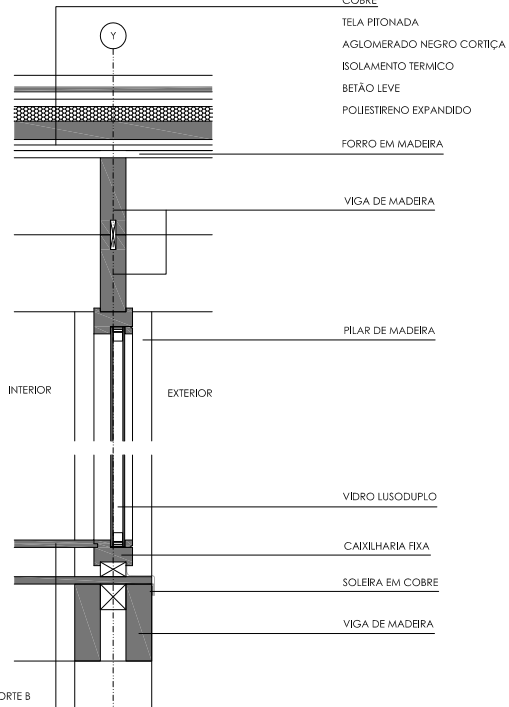
CORTE B
