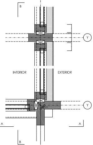
PLANTA
